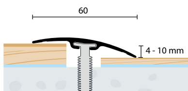
Prechodový profil 60x6,5 mm Výškový rozdiel 4-10 mm
