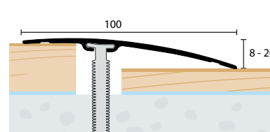
Prechodový profil 100x6,5 mm Výškový rozdiel 8-20 mm
