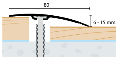
Prechodový profil 80x6,5 mm Výškový rozdiel 6-15 mm
